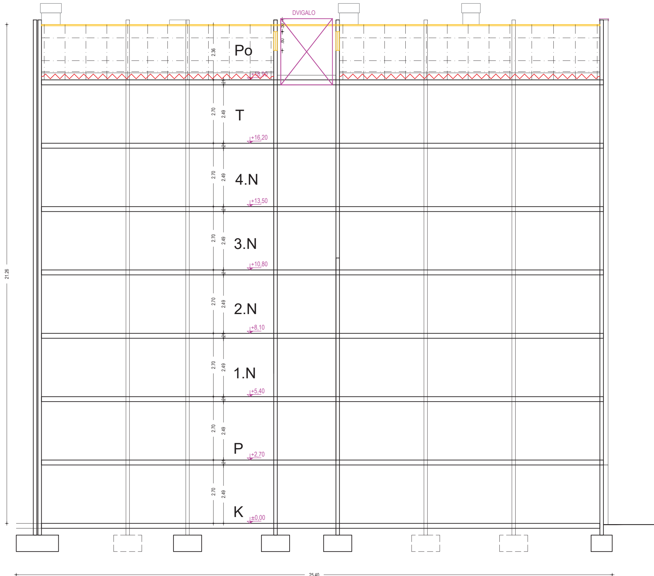
( Goriška 65_blok_15c ) PREREZ A-A - NOVO (ENERGETSKA SANACIJA) 1:100
