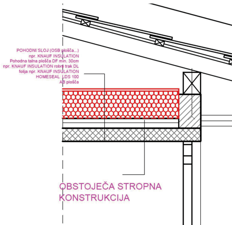
Detajl 4: Toplotna izolacija proti neogrevanemu podstrešju
