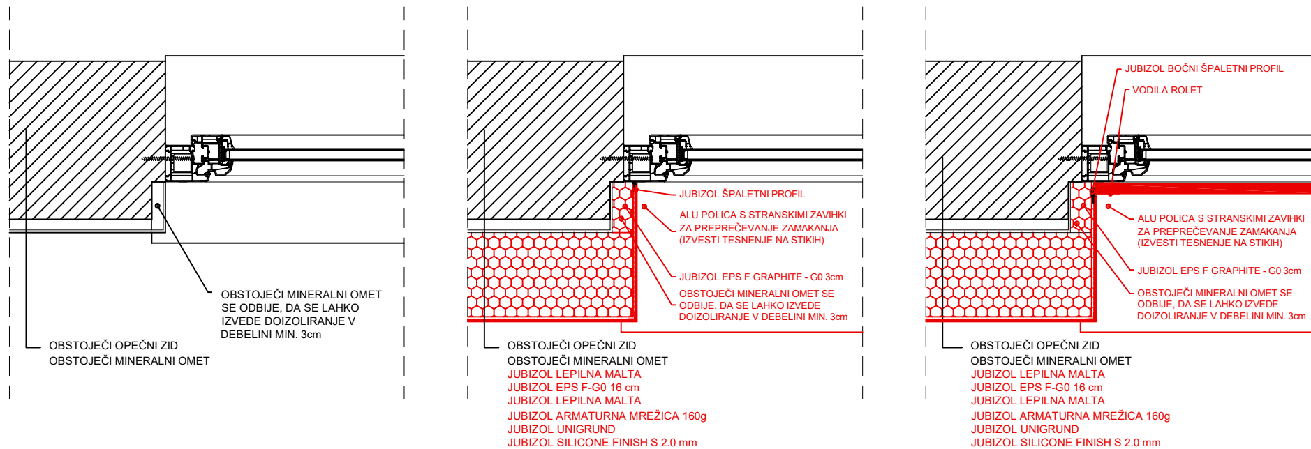
D2 - NOVO varianta brez izvedbe zunanjih rolet
