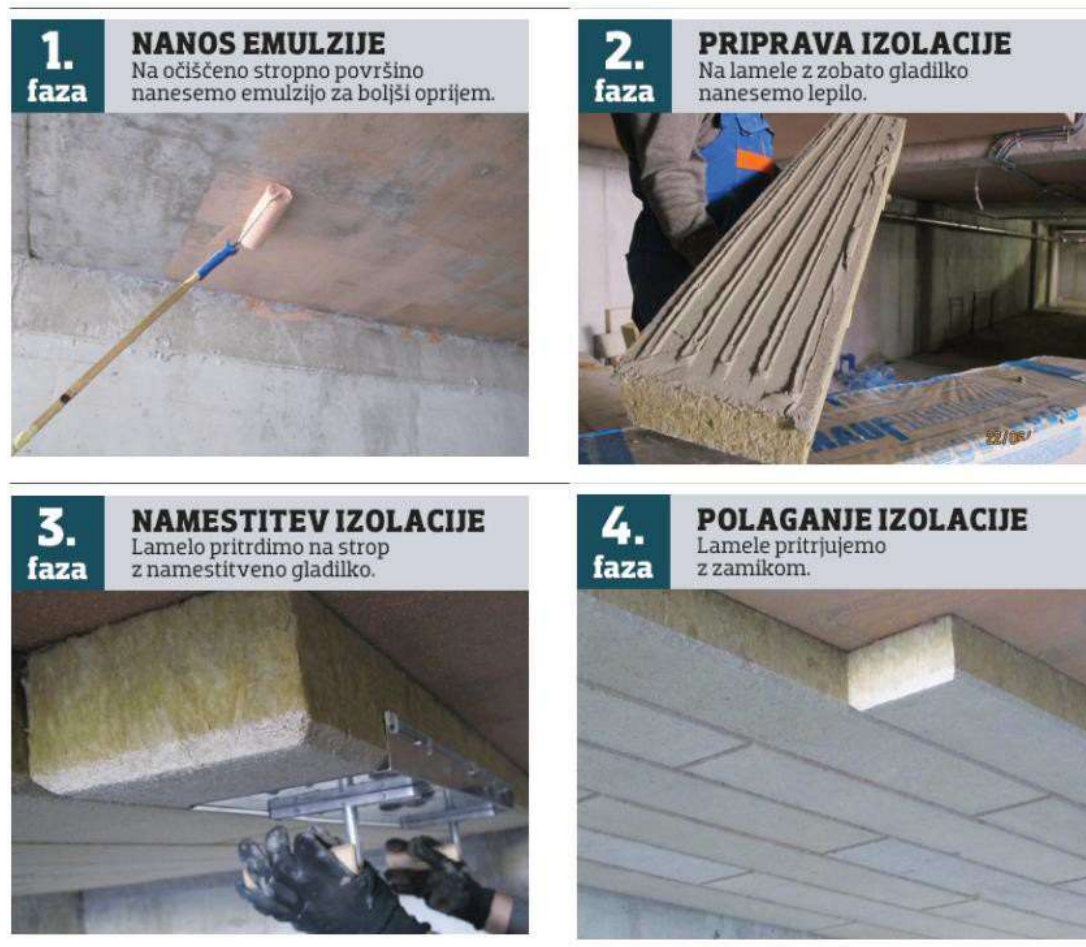
sliki – prikaz toplotne izolacije stropa kleti s ploščami CLT C1
