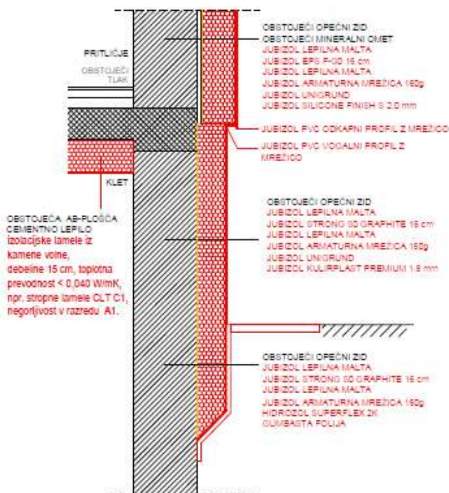
Skica 3: izvedba izolacije fasade stika s terenom
