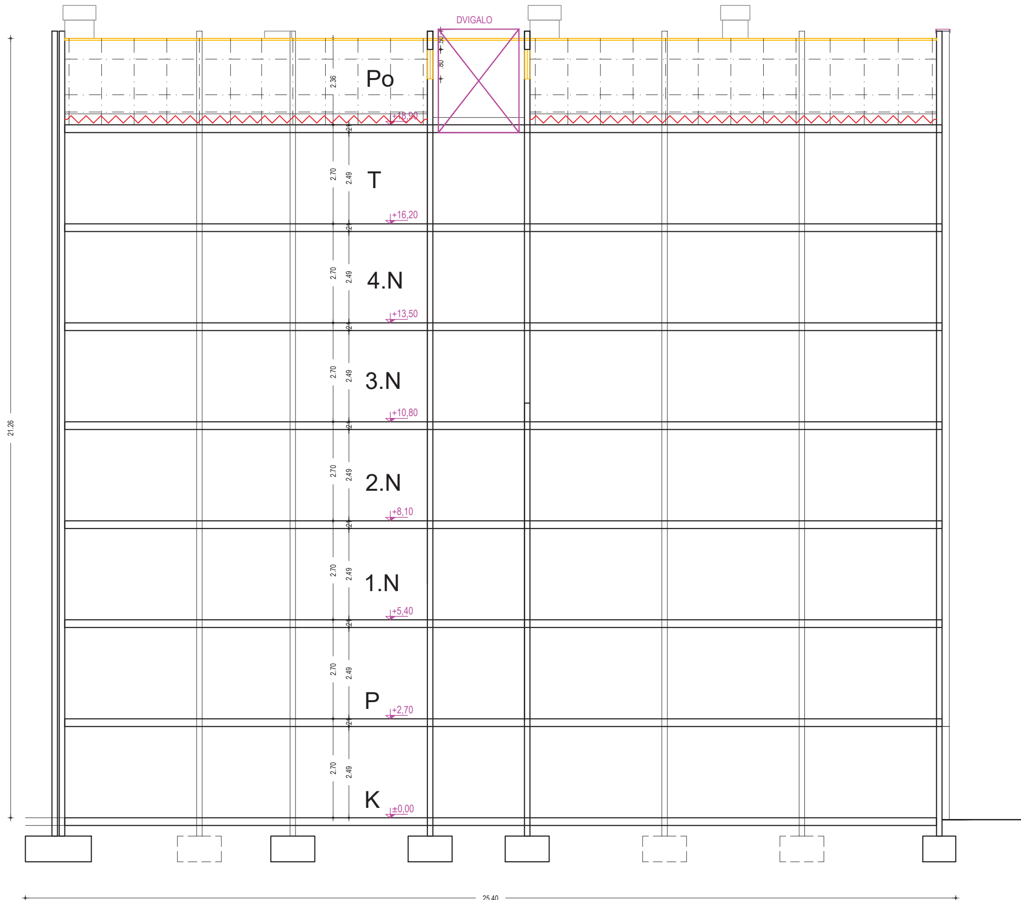
( Goriška 61_blok_13c ) PREREZ A-A - NOVO (ENERGETSKA SANACIJA) 1:100
