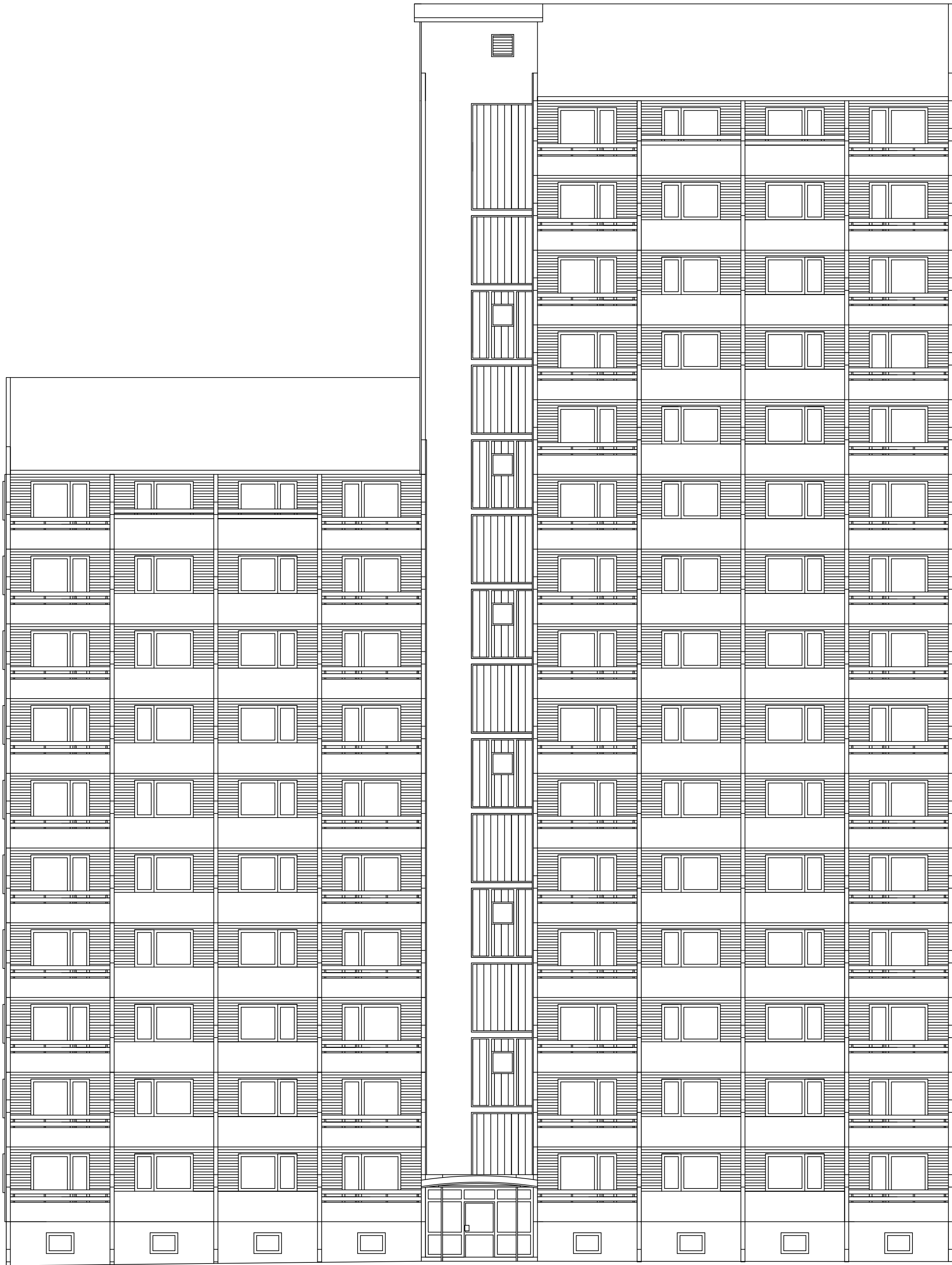
FASADA SEVEROVZHOD (obstoječe stanje)
