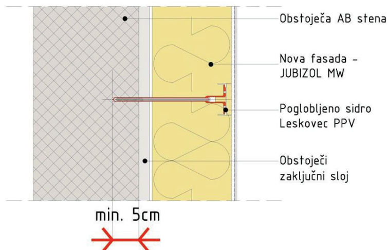
Detajl 1: poglobljeni sidri s pokrovčki iz izolacijskega materiala
