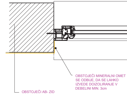
D2 - OBSTOJEČE STANJE
