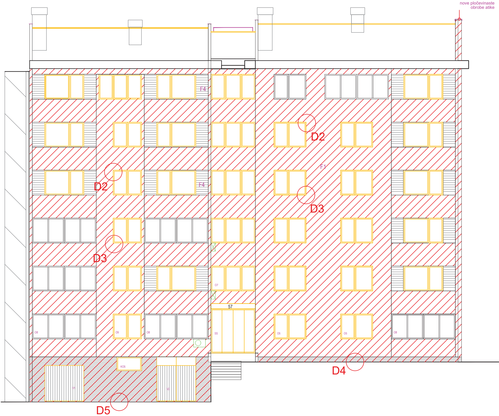
( Goriška 57_blok_11c ) FASADE - NOVO (ENERGETSKA SANACIJA) 1:100
